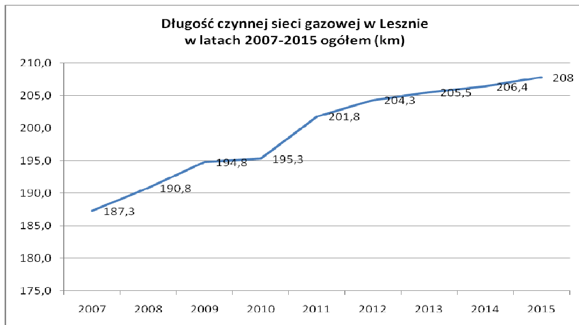
Wykres 61 Długość czynnej sieci gazowej w Lesznie w latach 2007-2015 ogółem (w kilometrach)
