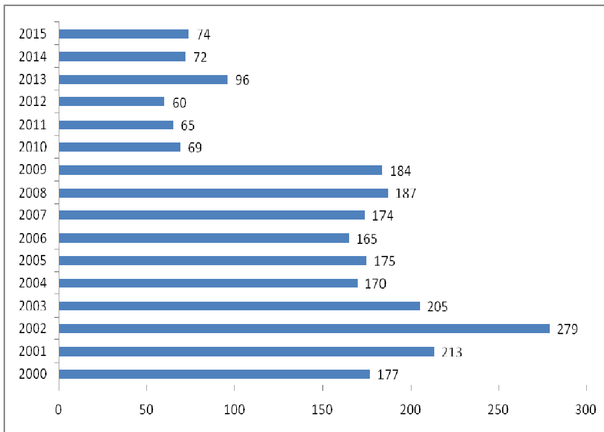
Wykres 56 Emisja zanieczyszczeń pyłowych powietrza z zakładów szczególnie uciążliwych w Lesznie w latach 2000-2015 (w t/r)
