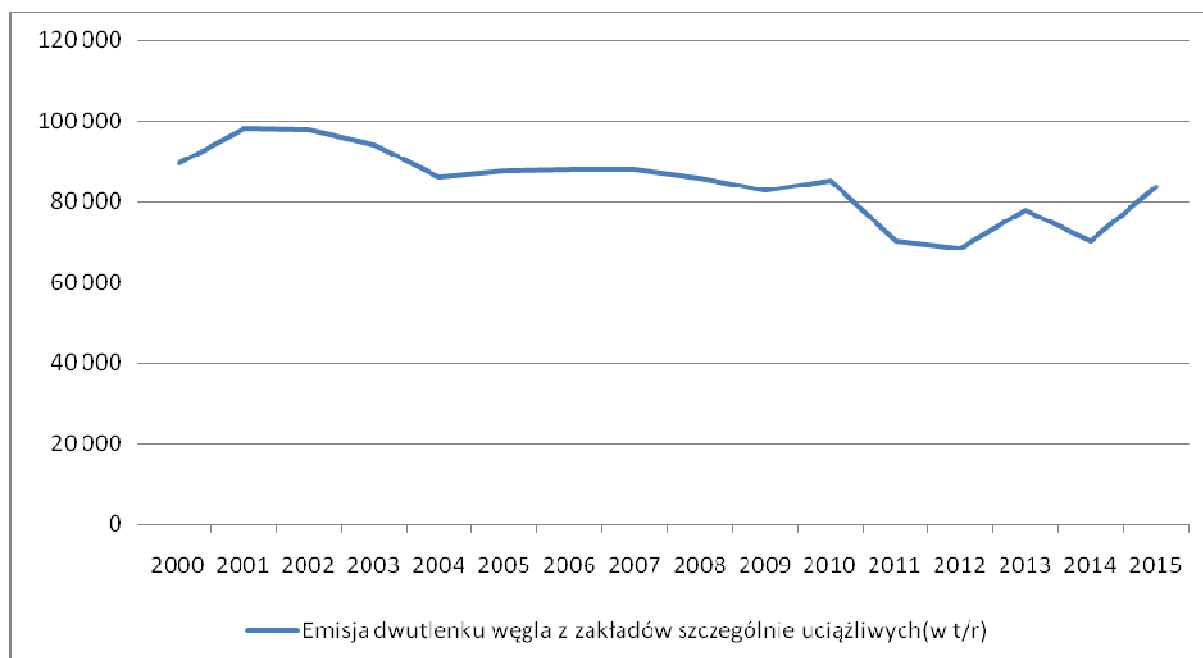
Wykres 55 Emisja dwutlenku węgla z zakładów szczególnie uciążliwych w Lesznie w latach 2000-2015 (w t/r)
