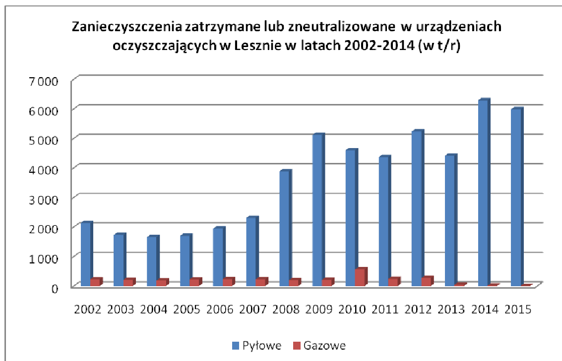
Wykres 57 Zanieczyszczenia zatrzymane lub zneutralizowane w urządzeniach oczyszczających w Lesznie w latach 2002-2015 (w t/r)
